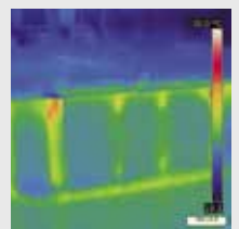
Verifica delle perdite di calore nel Nordic Insulation System
